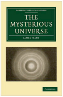
图 1 神秘的宇宙
